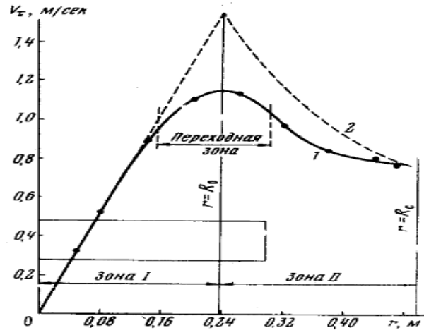
Рис. 1. Зависимость v_c от r : 1 — для сосуда с радиально-лопастной мешалкой, по данным работы [1]; d_m = 600 мм; D_c = 1000 мм; H_{ж} = D_c ; n = 63 об/мин; вода; 2 — расчет по модели вихря Ранкина
